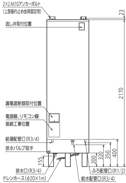
正面図
