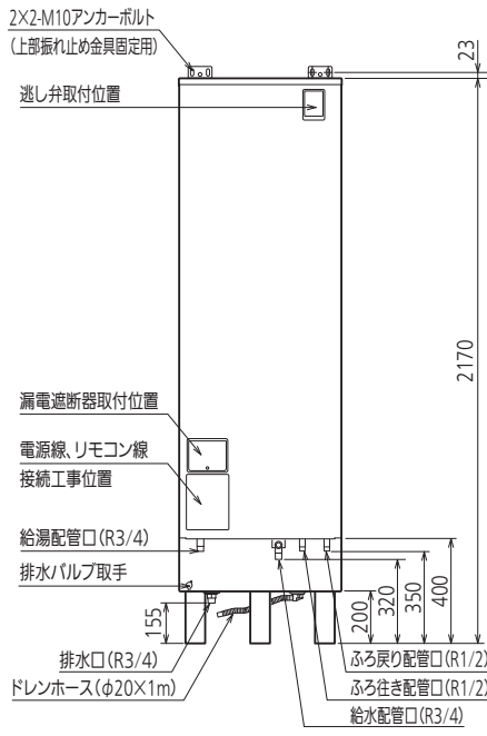
正面図
