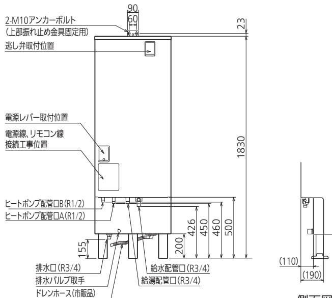
正面図
