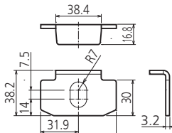
L型座金 (同梱部品)
