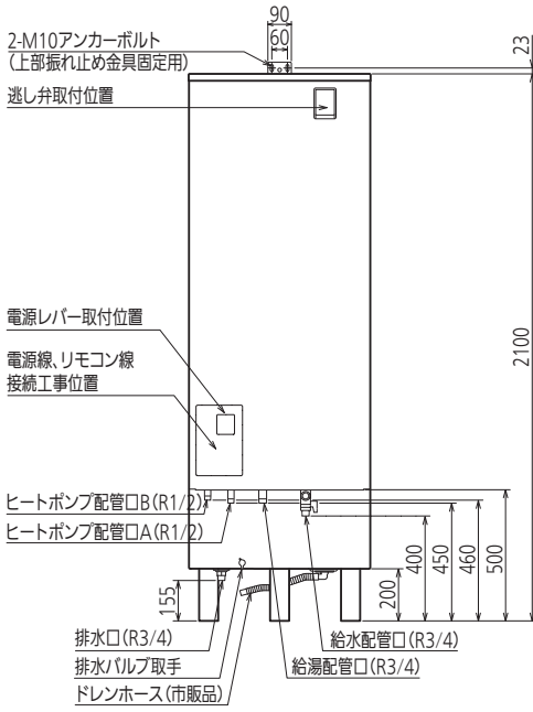
正面図
