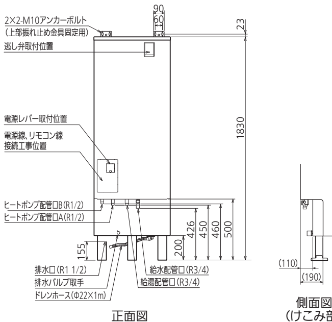
正面図
