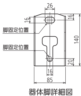
器体脚詳細図
