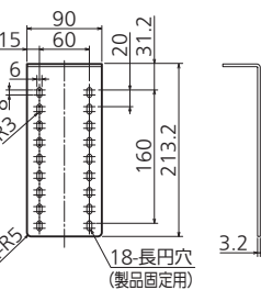
上部振れ止め金具 (同梱部品)
