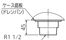
排水口寸法
