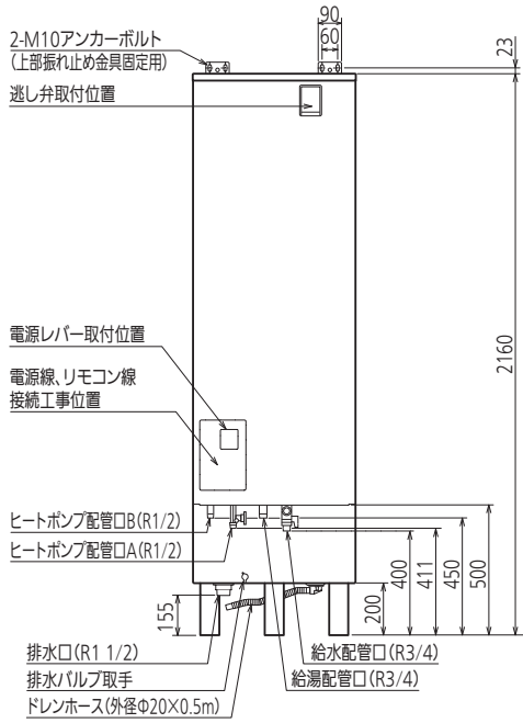
正面図
