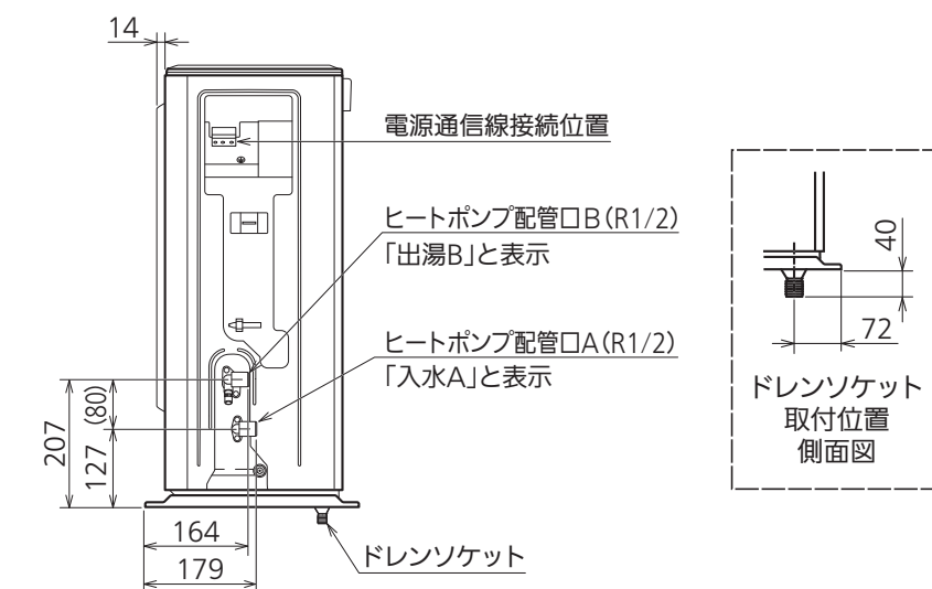
側面図
