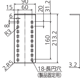
上部振れ止め金具 (同梱部品)
