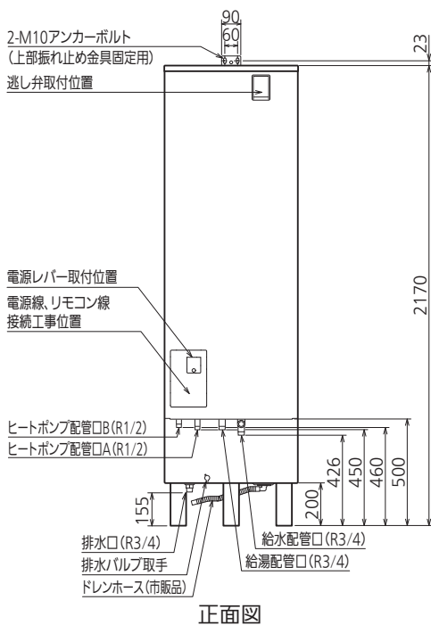
正面図
