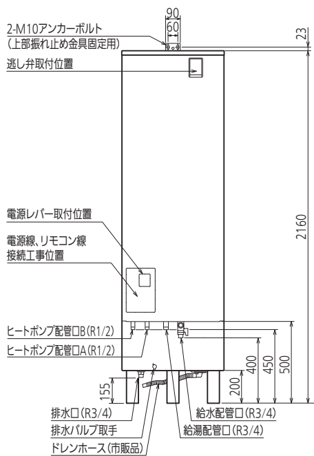
正面図
