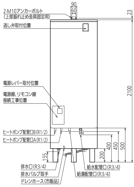
正面図
