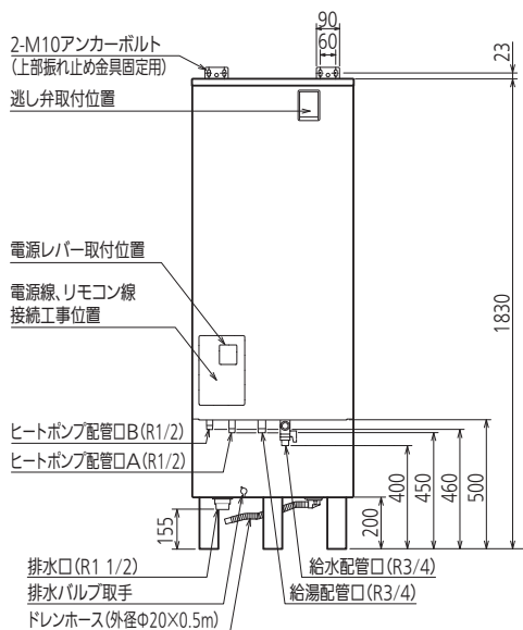
正面図
