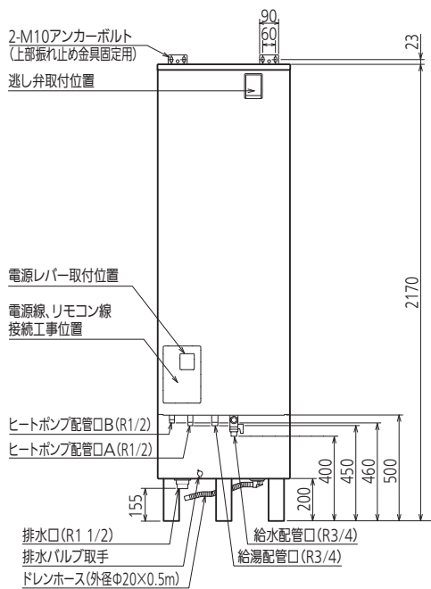
正面図
