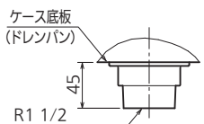
排水口寸法
