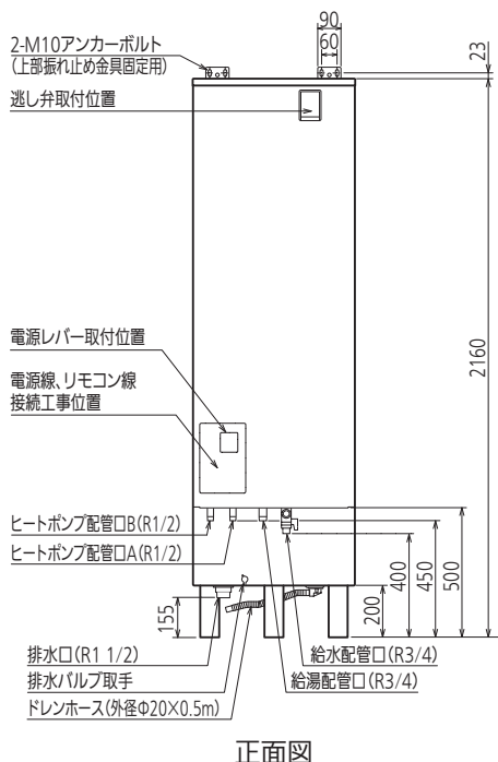
正面図
