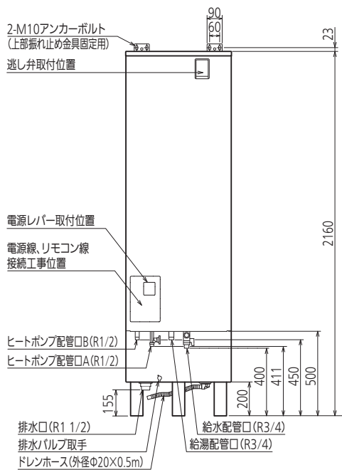
正面図
