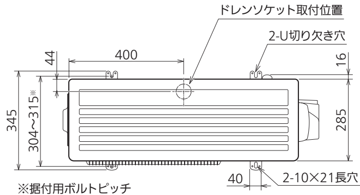
上面図
