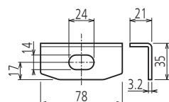
BWL型座金 (同梱部品)
