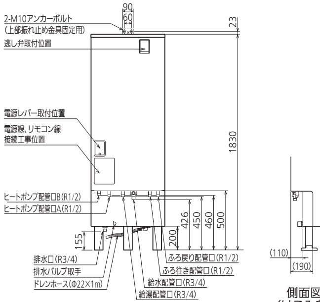
正面図
