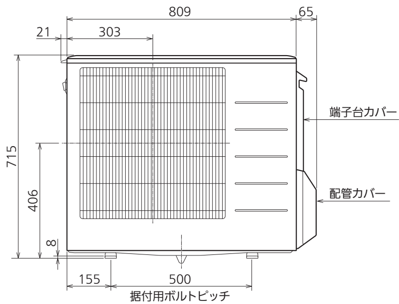
正面図
