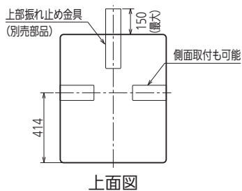
上面図
