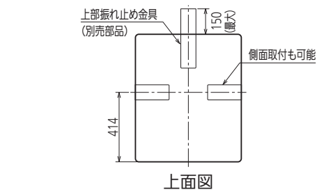
上面図
