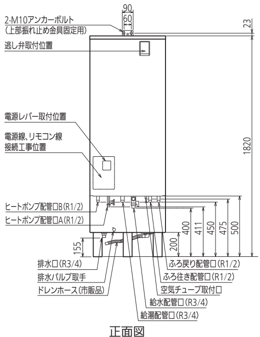
正面図
