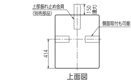
上面図
