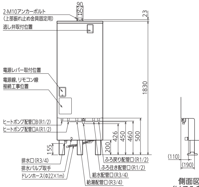
正面図
