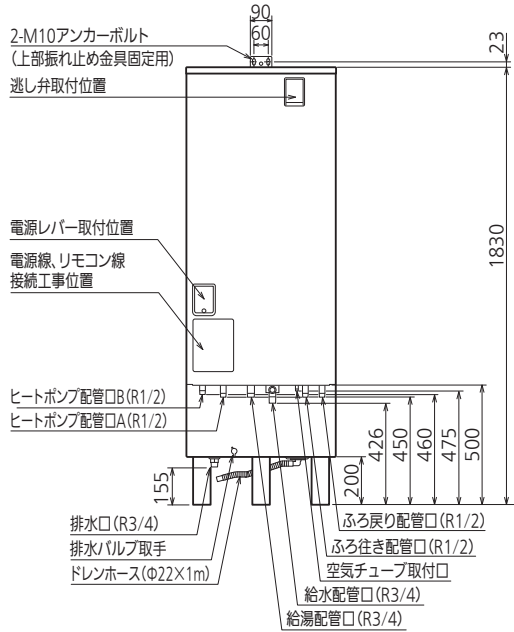
正面図
