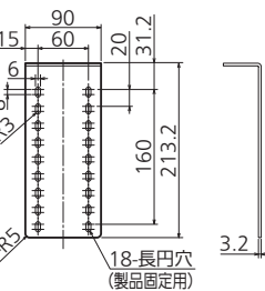
上部振れ止め金具 (別売部品)
