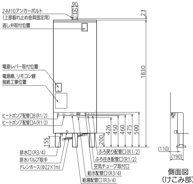
正面図
