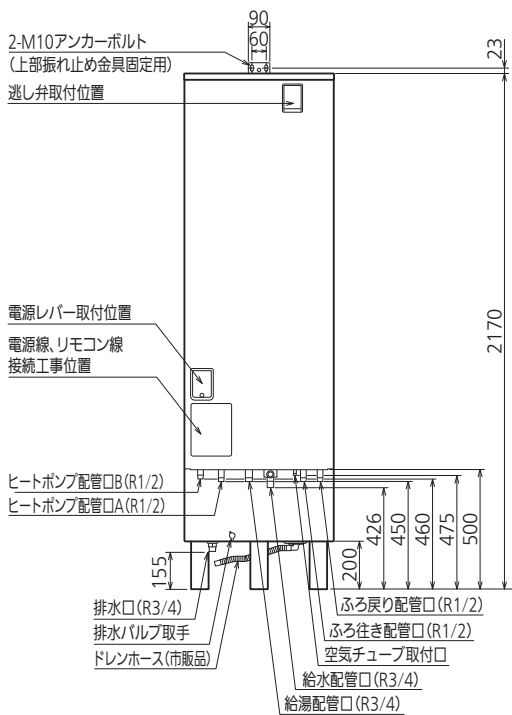
正面図
