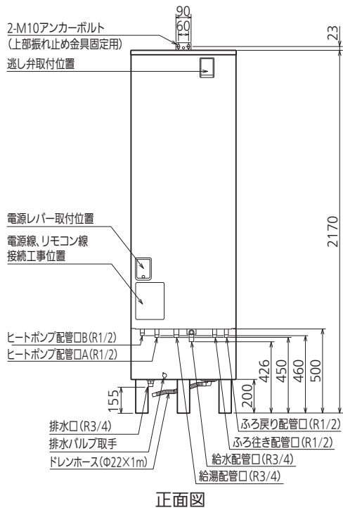
正面図
