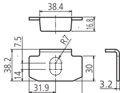
器体脚詳細図
