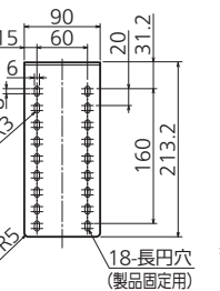
上部振れ止め金具 (別売部品)
