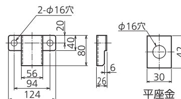
脚固定金具 (別売部品)
