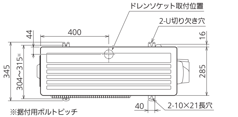
上面図
