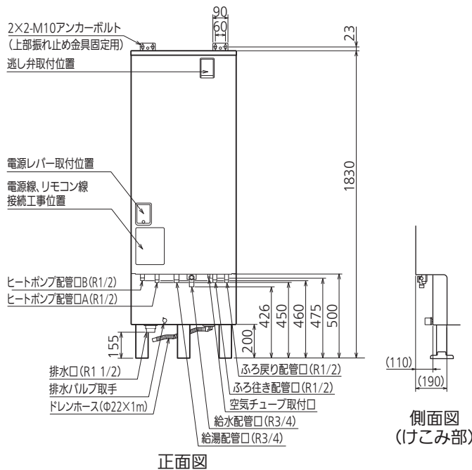
正面図
