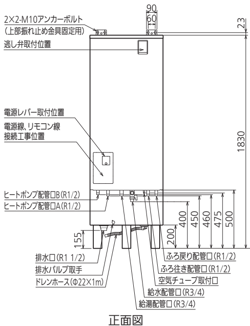
正面図
