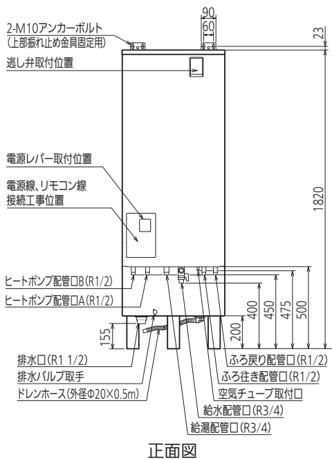
正面図
