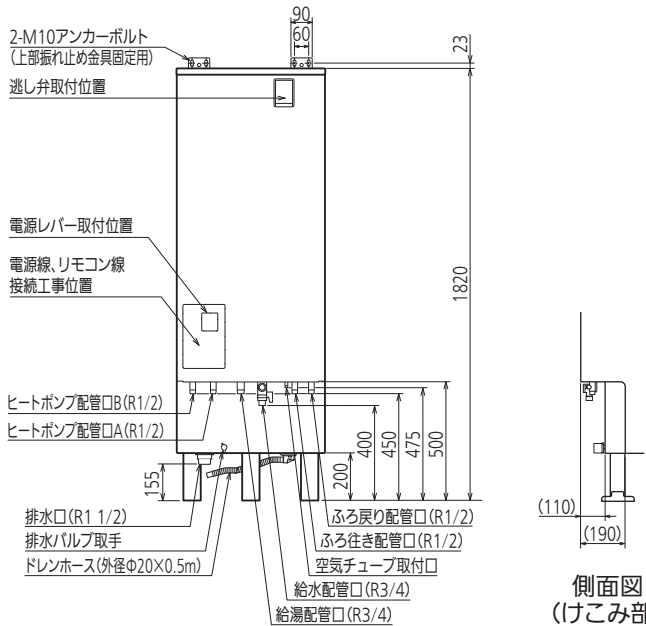
正面図
