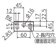
2-長円穴 (壁面固定用)
