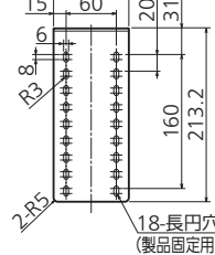
上部振れ止め金具 (同梱部品)
