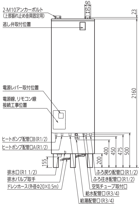
正面図
