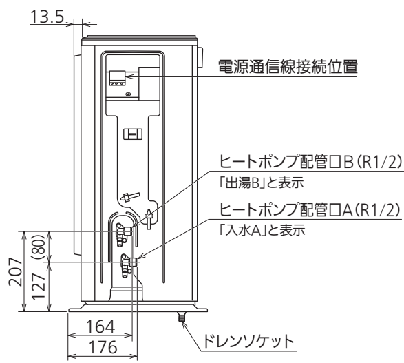
側面図
