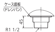
排水口寸法
