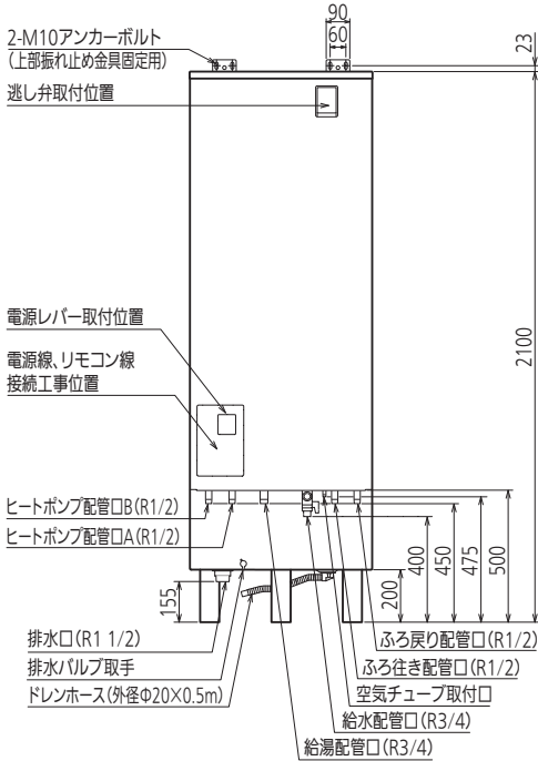
正面図
