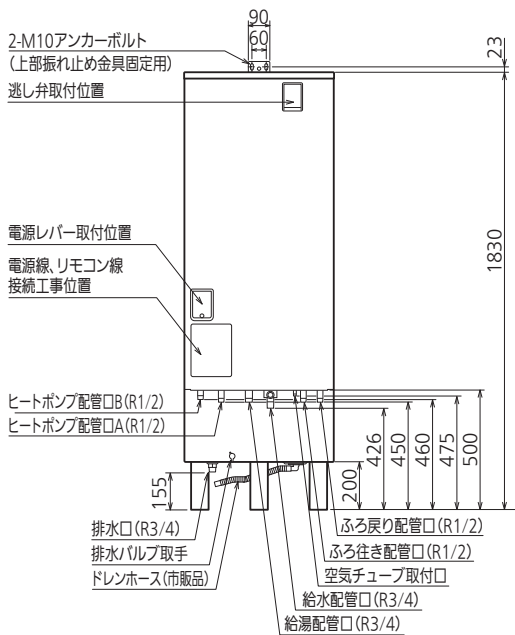
正面図
