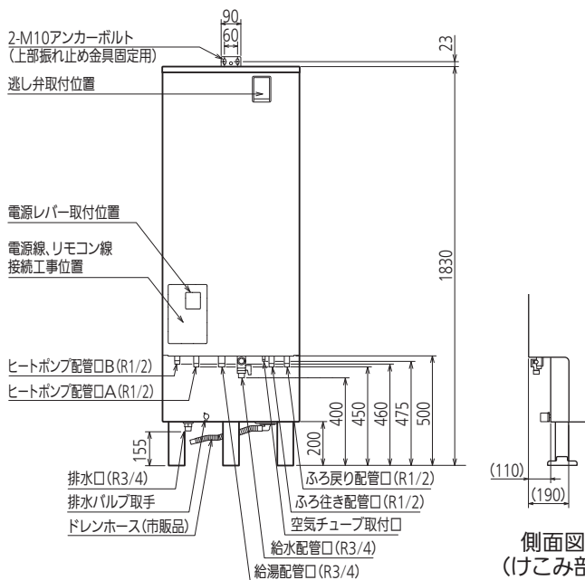
正面図
