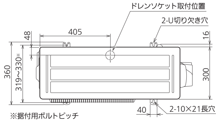
上面図
