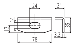
BWL型座金 (同梱部品)
