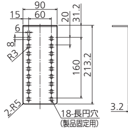
上部振れ止め金具 (別売部品)
