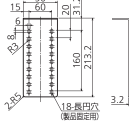
上部振れ止め金具 (別売部品)
