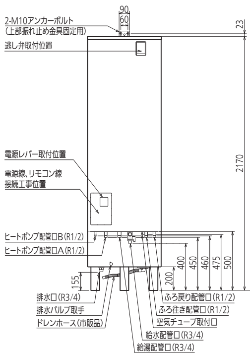
正面図
