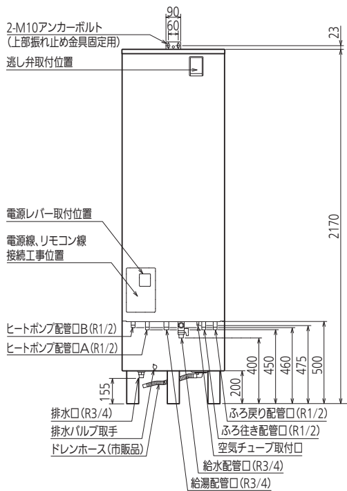
正面図
