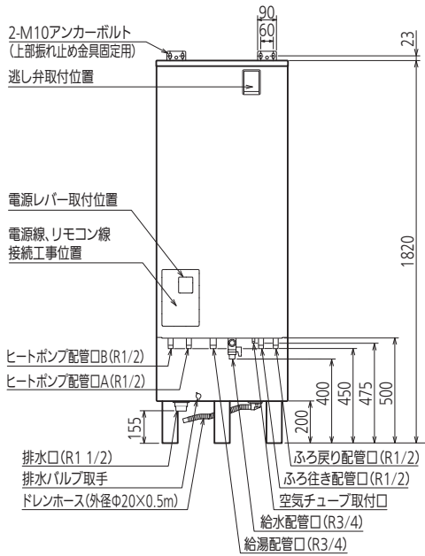
正面図
