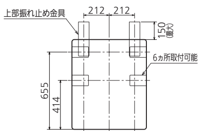
上面図
