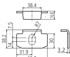
L型座金 (同梱部品)
