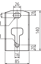
器体脚詳細図
