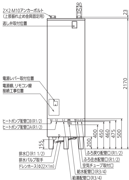
正面図
