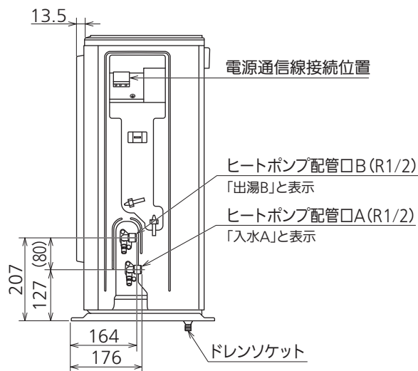
右側面図
