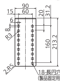
上部振れ止め金具 (同梱部品)
