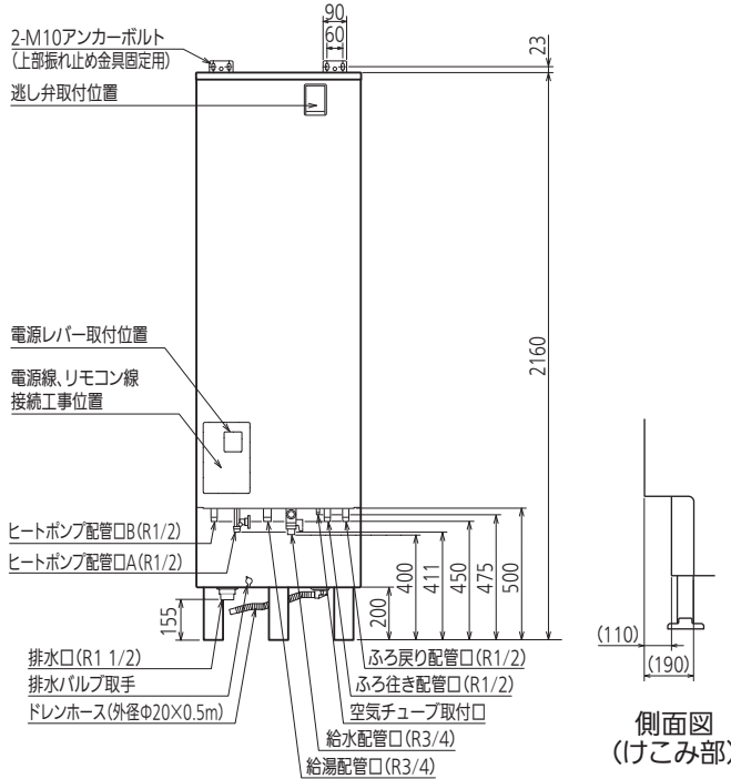
正面図
