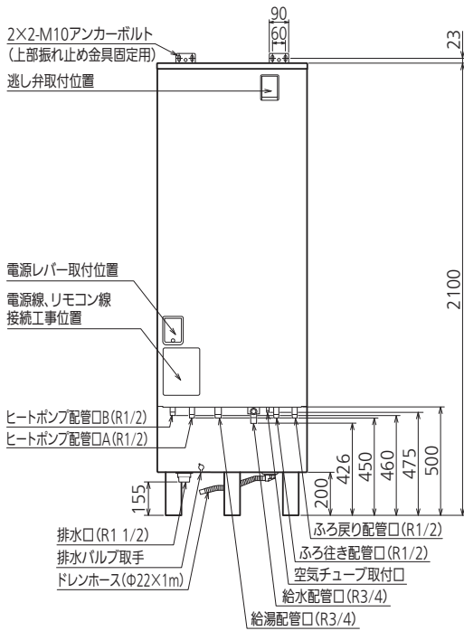
正面図
